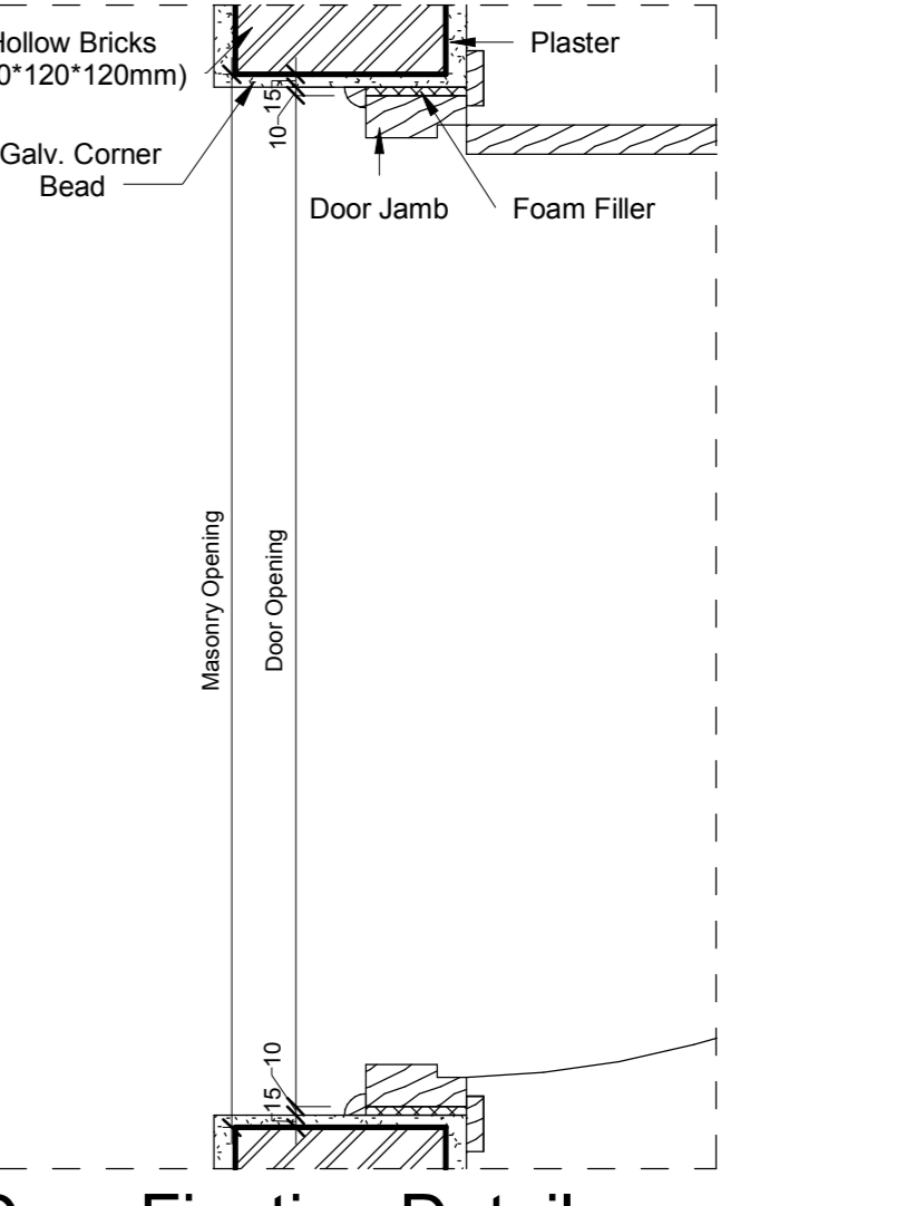
14 Door Fixation Detail 1 : 10
