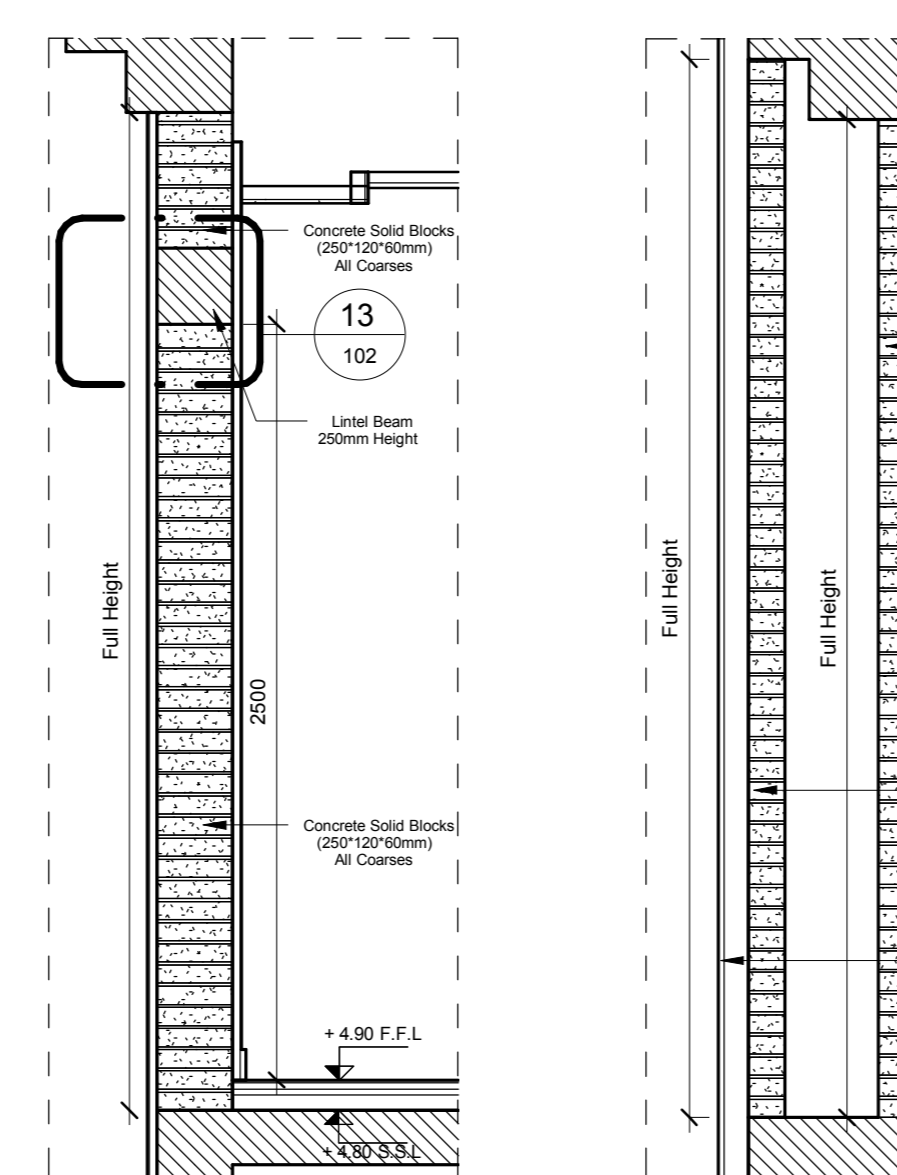
5 BW1 1 : 25
