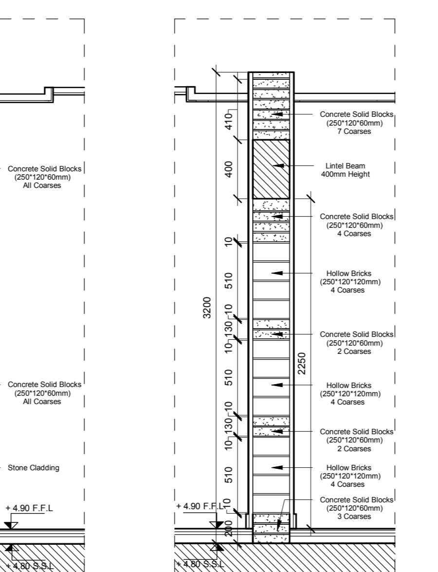
6 BW2 1 : 25
