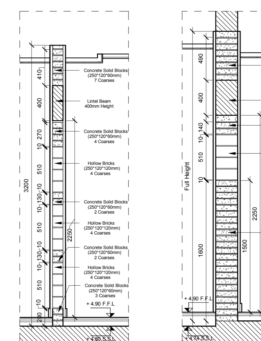
7 BW3 1 : 25
