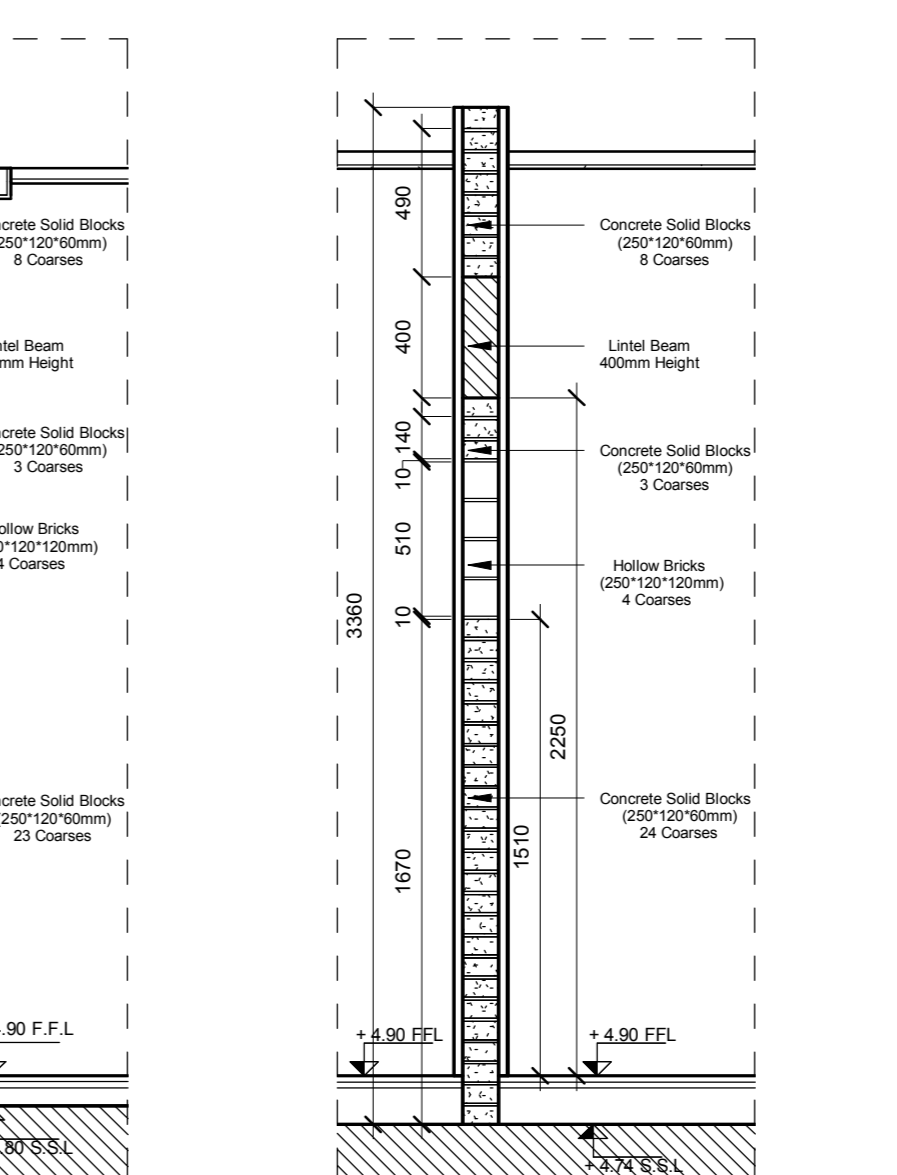
8 BW4 1 : 25
