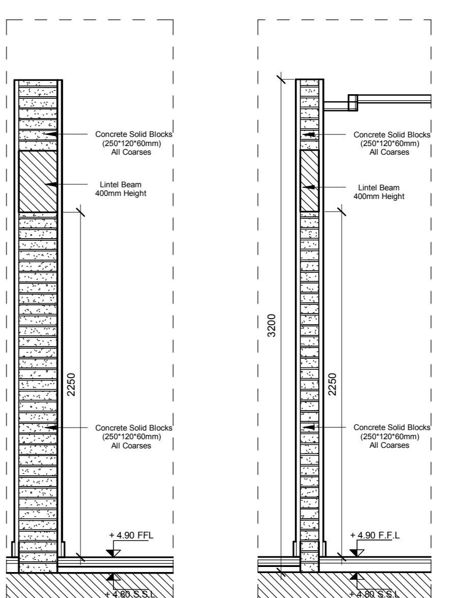
9 BW5 1 : 25
